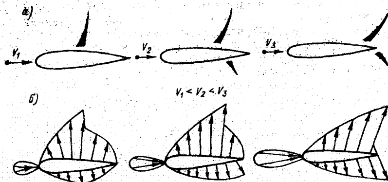
Рис. 1.9. Изменение характера распределения давления при увеличении скорости: а – перемещение скачка уплотнения, б – диаграммы распределения давлений.
