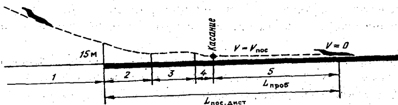
Рис. 3.6. Этапы посадки самолета.
