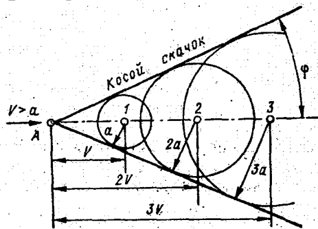
Рис. 1.11. Косой скачок уплотнения.
