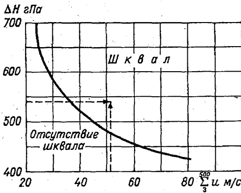
Рис. 7.7. График для определения возможности шквала.
