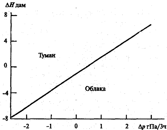
Рис. 9.15. График для определения возможности перехода низкой облачности в туман, используемый в Ашхабаде.
