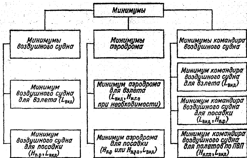
Рис. 9.1. Схема видов минимумов погоды для авиации.
