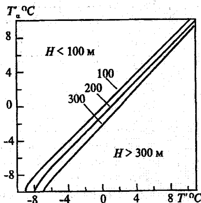
Рис. 9.12. График для прогноза высоты нижней границы облаков по прогностическим значениям температуры T' и температуры точки росы T'_d .
