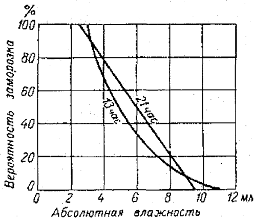
Рис. 6.10. График Михельсона для определения вероятности заморозков.
