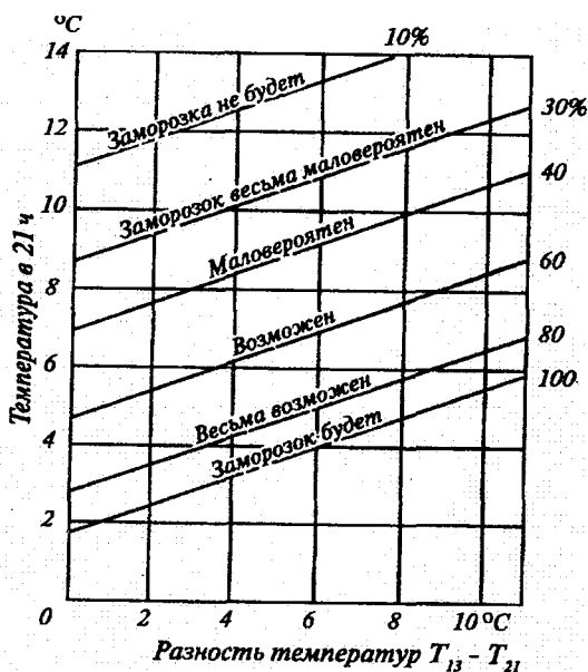
Рис. 6.11. График Броунова для определения вероятности заморозков.
