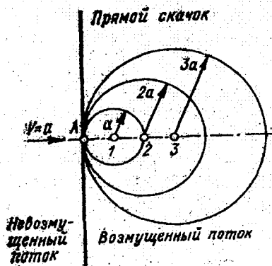
Рис. 1.10. Прямой скачок уплотнения.
