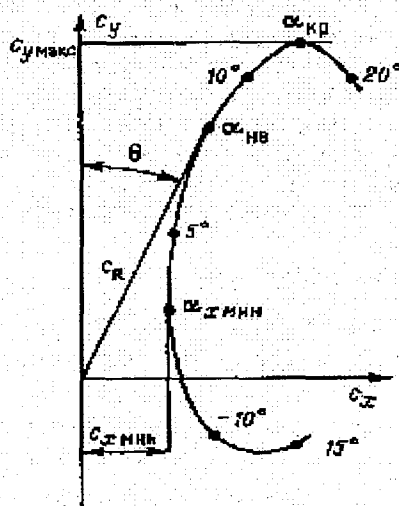
Рис. 1.6. Поляра крыла самолета.
