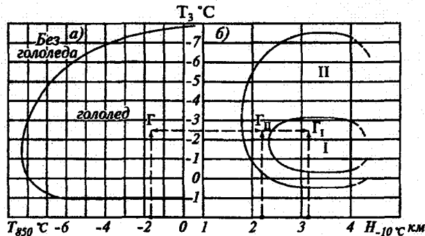
Рис. 10.3. Номограмма Р.А. Ягудина для определения возможности возникновения гололеда (а) и его интенсивности (б): I – зона умеренного гололеда; II – зона слабого гололеда.
