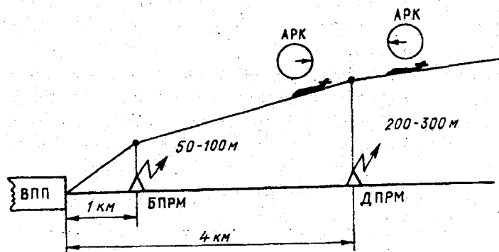
Рис. 4.2. Примерная схема работы радиотехнических средств навигации.
