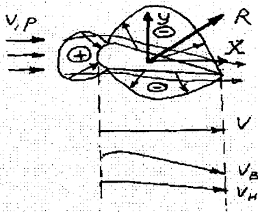
Рис. 1.4. Обтекание крыла потоком при \alpha > 0 .
