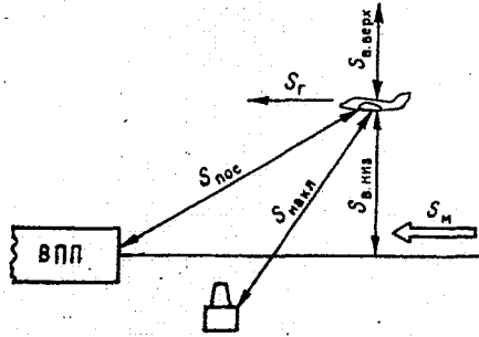
Рис. 9.2. Характеристики видимости, используемые при метеорологическом обеспечении полетов.
