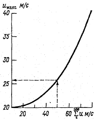
Рис. 7.8. Определение максимальной скорости ветра при шквале.
