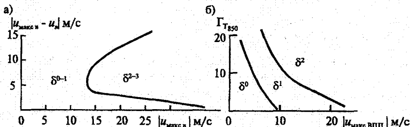
Рис. 8.8. Графики для прогноза болтанки в приземном слое: а – по приземным данным; б – по данным о ветре на ВПП и горизонтальном градиенте температуры на уровне 850 гПа.
