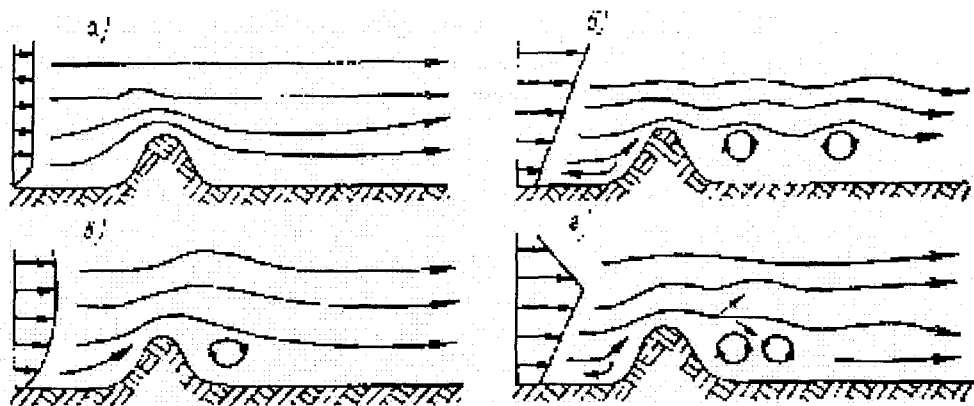
Рис. 8.4. Структура воздушного потока над горами.
