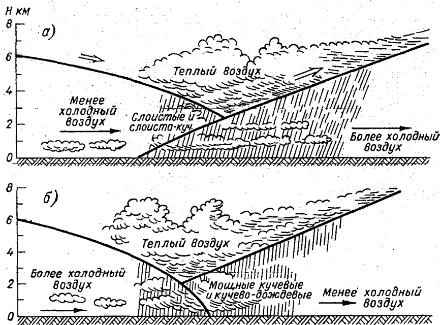
Рис. 9.7. Схема облачной системы фронтов окклюзии по типу теплого (а) и по типу холодного (б).
