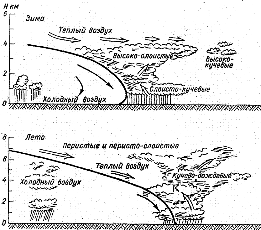
Рис. 9.6. Схема облачной системы холодного фронта второго рода.
