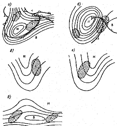
Рис. 8.6. Распределение и положение зон болтанки при различных типах синоптических ситуаций:
