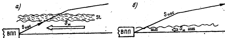
Рис. 9.3. Метеорологические ситуации, приводящие к различию между посадочной и метеорологической видимостью:
