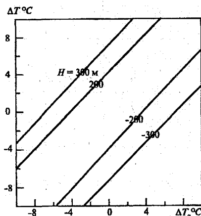
Рис. 9.13. График для оценки изменений высоты нижней границы облаков.
