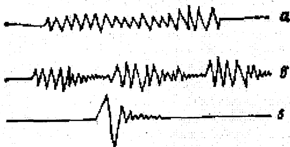
Рис. 8.2. Вид записей акселерографа при полете ВС в зонах турбулентности: а – непрерывная турбулентная зона; б – прерывистая турбулентная зона; в – отдельные толчки (броски) самолета.
