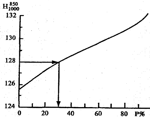
Рис. 10.2. График для определения вероятности возникновения гололеда.
