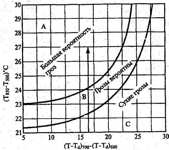
Рис. 11.1. График для прогноза гроз по методу Бейли.
