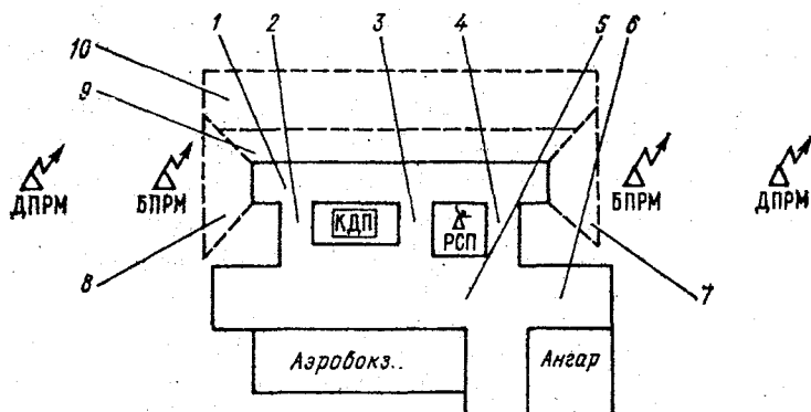
Рис. 4.1. Схема аэродрома (вариант):
