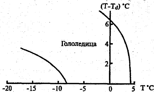
Рис. 10.4. График для прогноза гололедицы.
