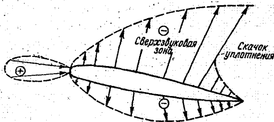
Рис. 1.8. Распределение избыточного давления при смешанном обтекании.
