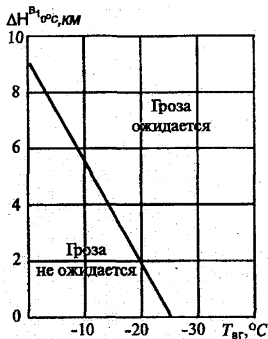
Рис. 11.3. График для прогноза гроз (по методу Г.Д. Решетова).
