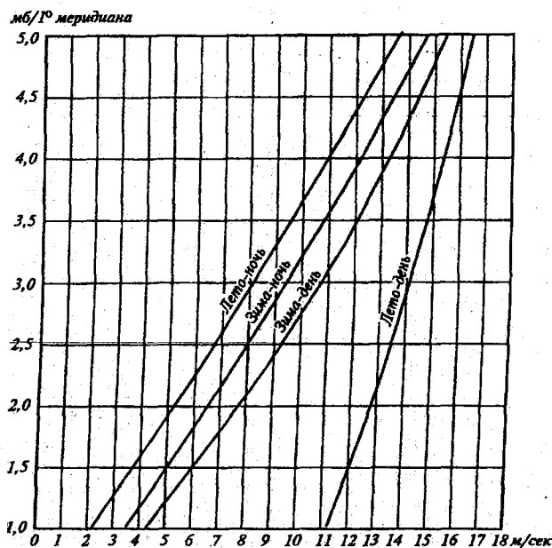
Рис. 7.5. График зависимости скорости ветра от горизонтального градиента давления.
