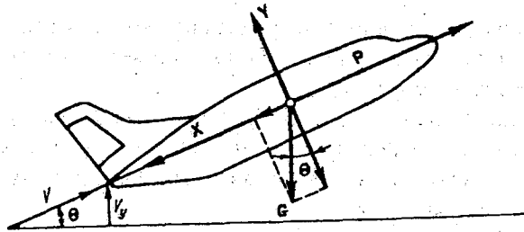
Рис. 3.2. Схема сил, действующих на самолет при подъеме.
