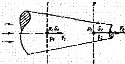
Рис. 1.1. Схема движения воздуха в трубке переменного сечения.
