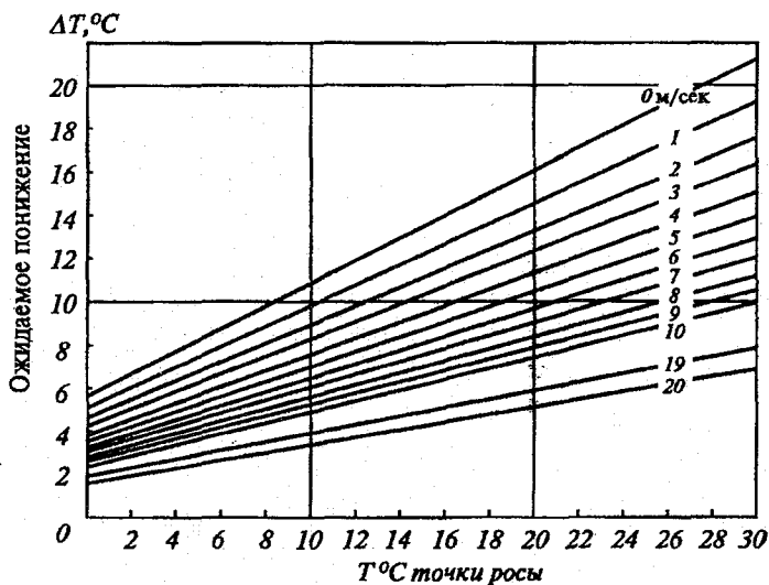
Рис. 6.7. Номограмма для определения ночного понижения температуры по данным наблюдений в 13 ч.
