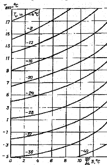
Рис. 11.2. График для определения температуры нулевого испарения.
