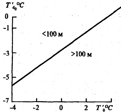
Рис. 9.14. График 3.А. Спарышкиной для прогноза облачности высотой до 100 м.
