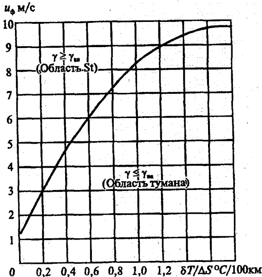
Рис. 9.21. График для прогноза адвективного тумана (по И.В. Кошеленко).
