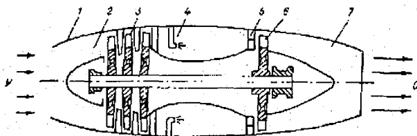
Рис. 6.3. Принципиальная схема турбореактивного авиационного двигателя: 1 – корпус; 2 – воздухозаборник; 3 – компрессор; 4 – камера сгорания; 5 – сопловый аппарат; 6 – турбина; 7 – реактивное сопло.
