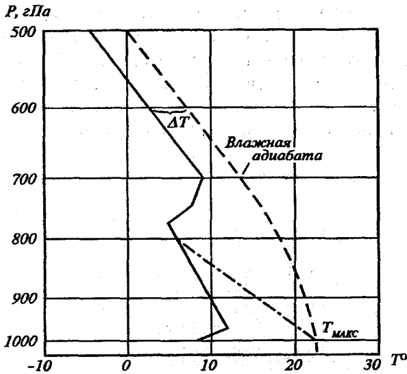
Рис. 7.6. График для прогноза максимальных порывов ветра у земли при грозах.
