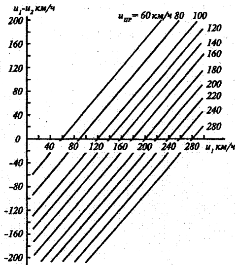
Рис. 7.16. Номограмма для прогноза скорости ветра на высотах на 24 ч (по методу Э.С. Ильиной).
