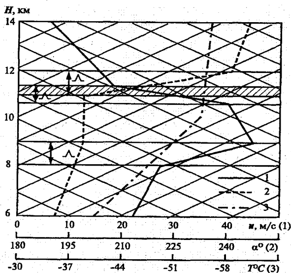
Рис. 8.7. Графический метод прогноза болтанки самолетов.
