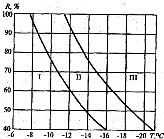
Рис. 9.24. График для прогноза туманов испарения.
