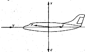
Рис. 3.1. Схема сил, действующих на самолет в горизонтальном полете.
