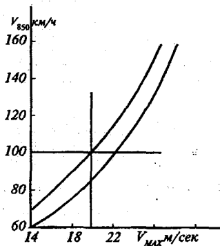
Рис. 7.11. График для прогноза скорости ветра у земли по данным о ветре на уровне 850 гПа.
