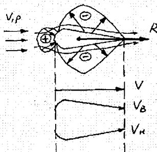
Рис. 1.3. Обтекание крыла потоком при \alpha = 0 .
