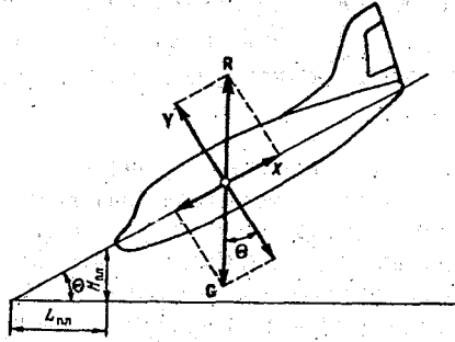
Рис. 3.3. Схема сил, действующих на самолет при планировании.
