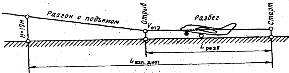
Рис. 3.4. Этапы взлета самолета.
