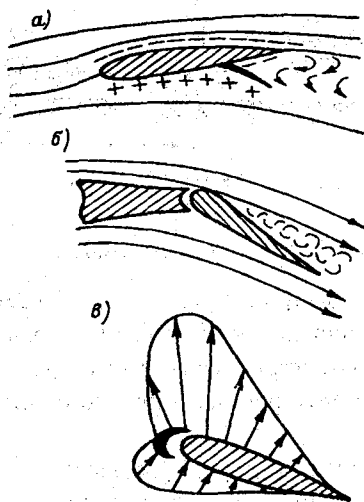
Рис. 3.5. Основные виды механизации крыла: а – щиток, б – закрылок, в – предкрылок.
