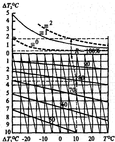
Рис. 9.20. Номограмма Б.В. Кирюхина для определения величины \Delta T_T .
