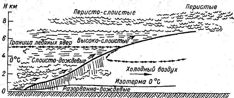
Рис. 9.4. Схема облачной системы теплого фронта.
