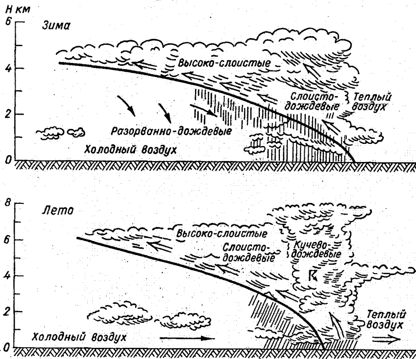
Рис. 9.5. Схема облачной системы холодного фронта первого рода.
