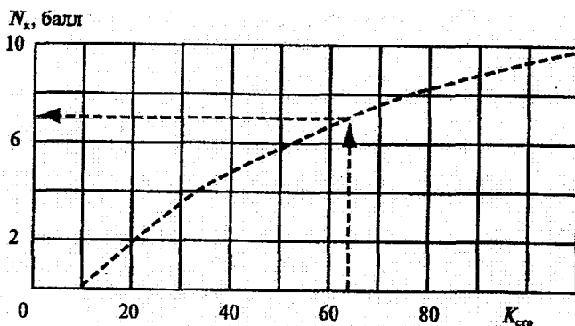
Рис. 9.8. Зависимость количества конвективной облачности от коэффициента стратификации.
