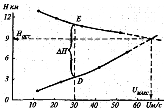
Рис. 7.17. Определение параметров струйного течения (по методу Е. Рейтера).
